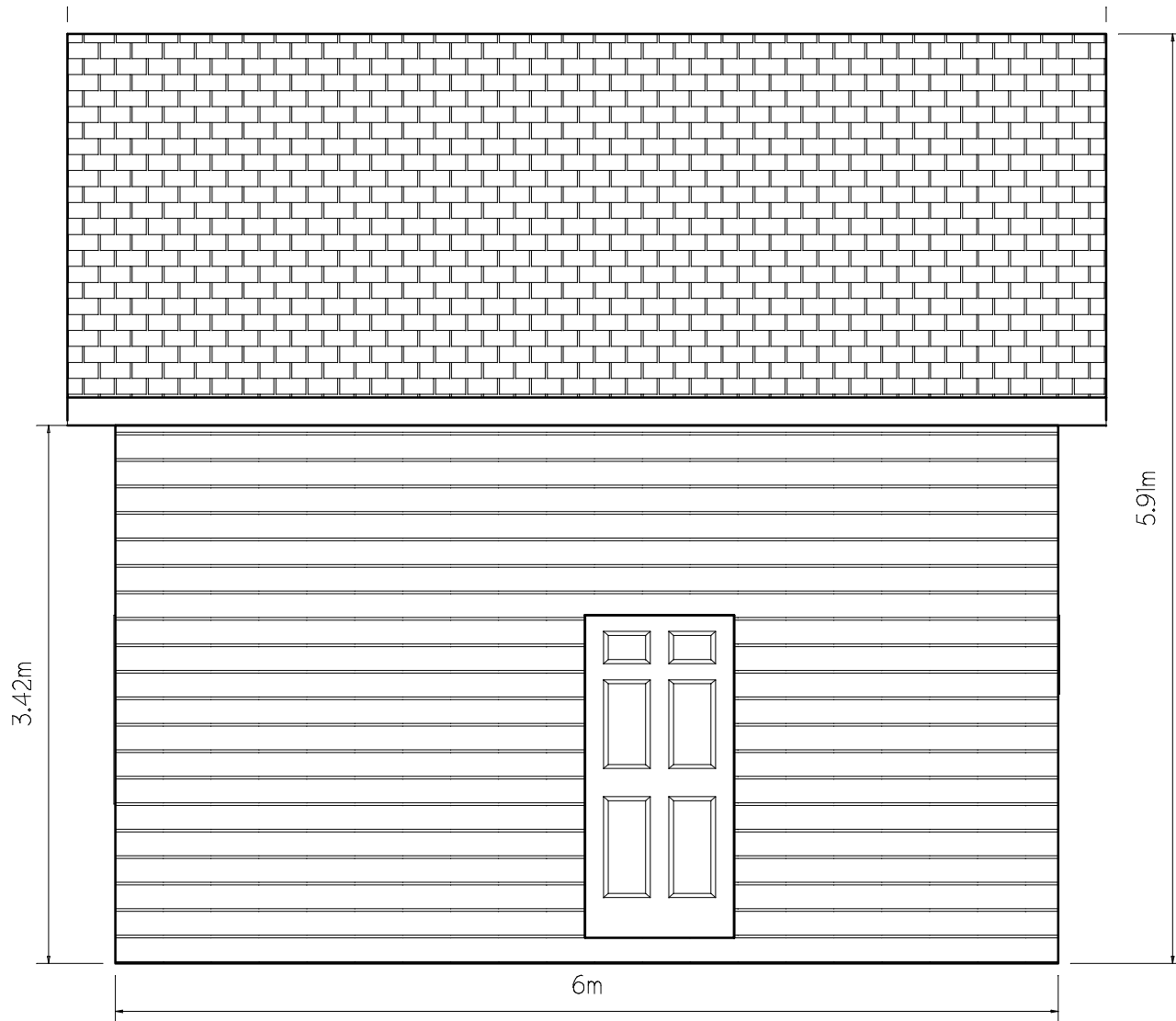
Вид справа
