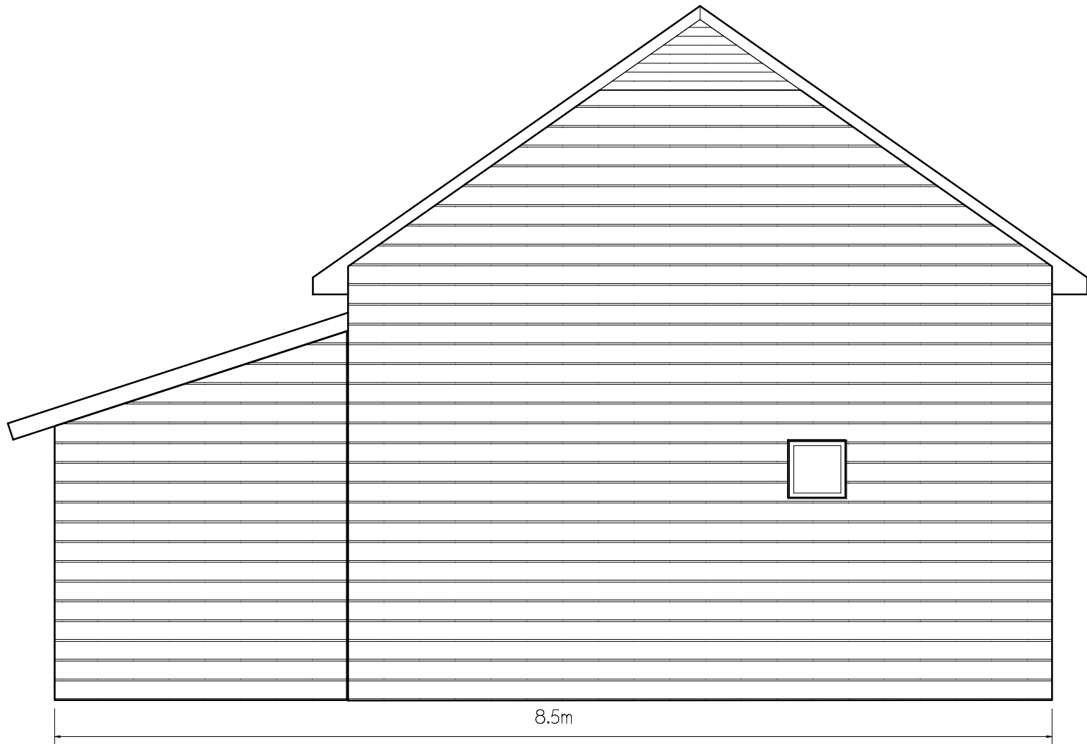
Вид сзади
