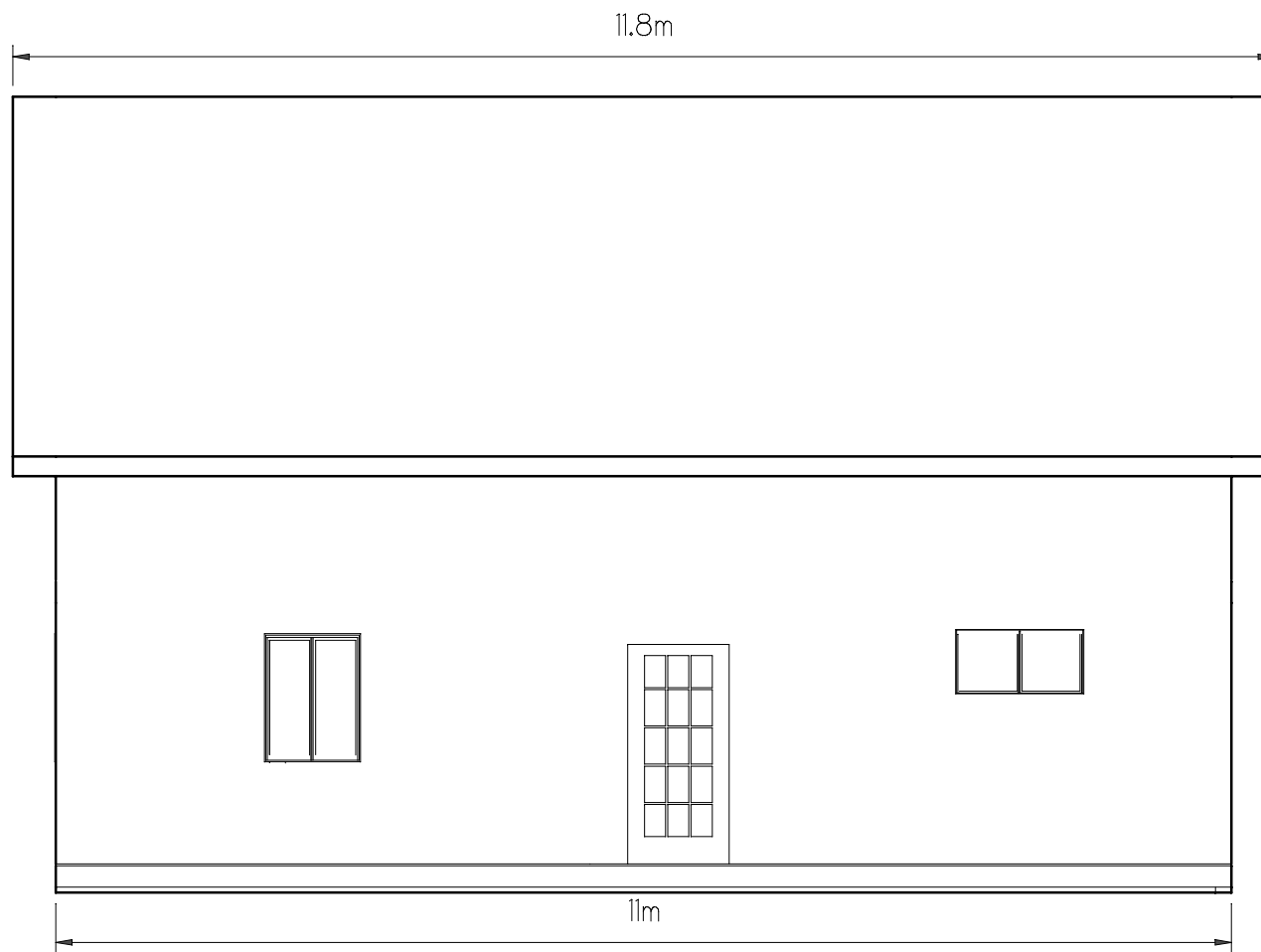
Вид справа
