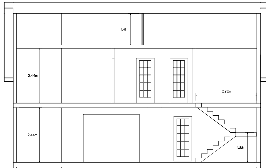
Разрез
