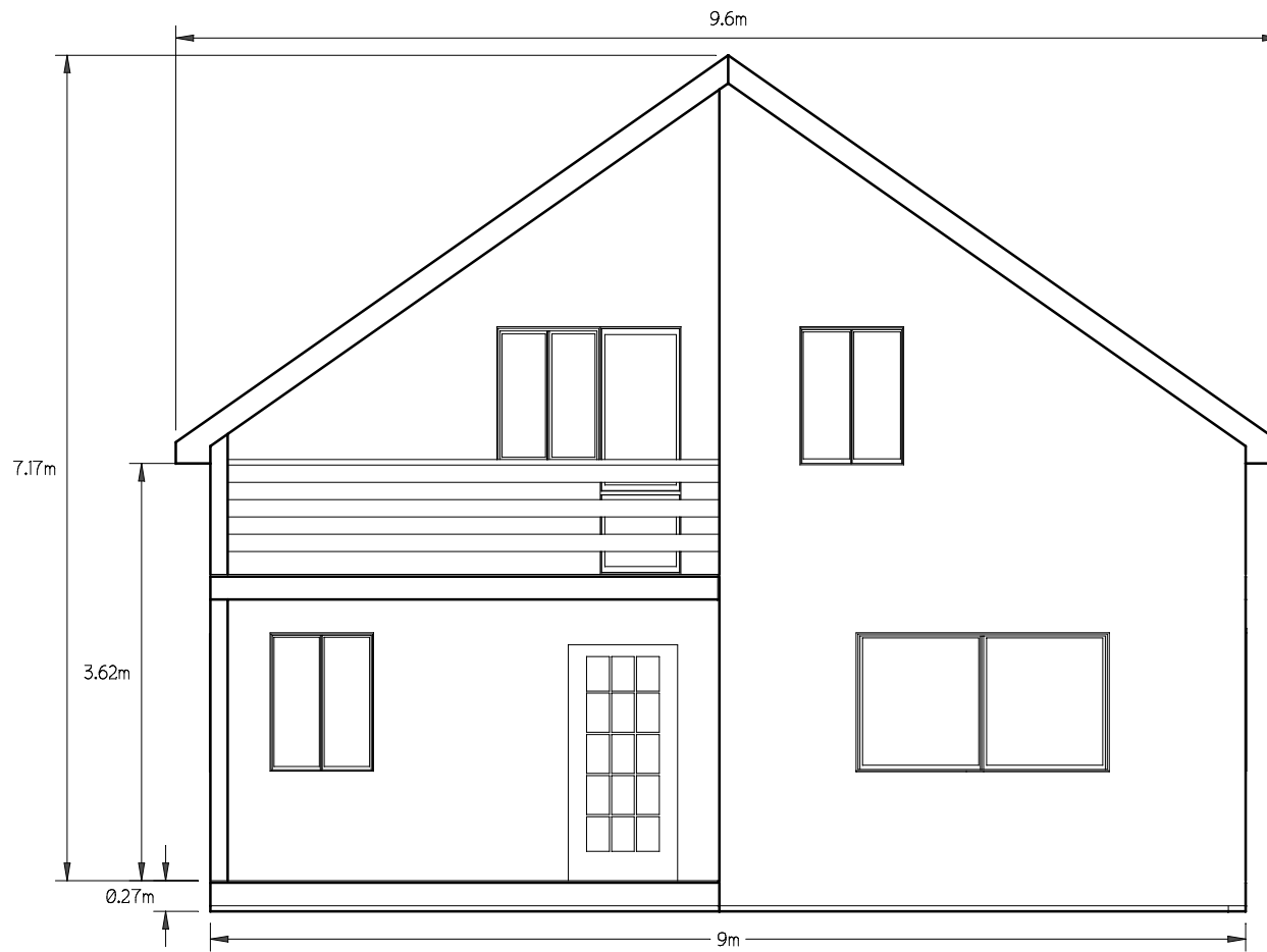
Вид спереди
